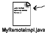
MyRemoteImpl.java
